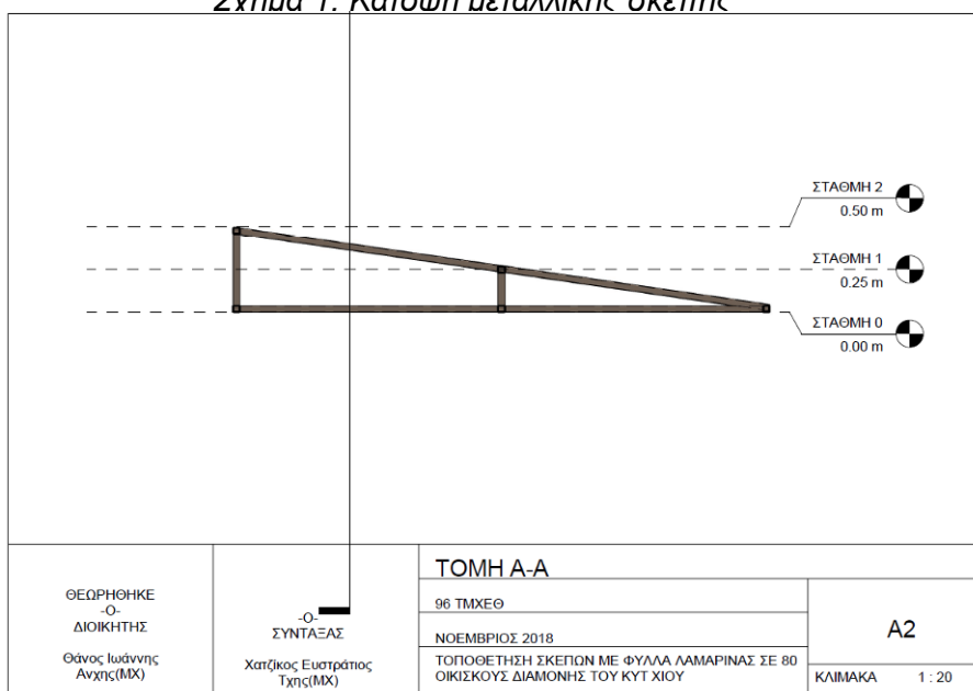
Σχήμα 2: Τομή Α-Α μεταλλικής σκεπής
