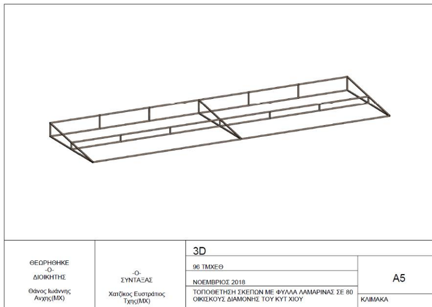
Σχήμα 5: Τρισδιάστατη απεικόνιση μεταλλικής σκεπής
