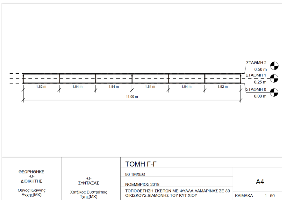
Σχήμα 4: Τομή Γ-Γ μεταλλικής σκεπής
