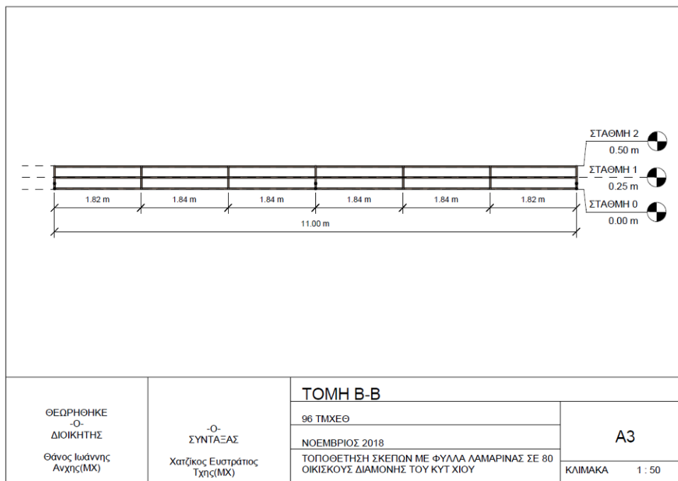
Σχήμα 3: Τομή Β-Β μεταλλικής σκεπής
